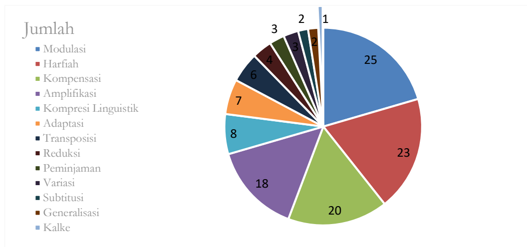
Gambar 21. Diagram Frekuensi Penggunaan Teknik Penerjemahan sebagai berikut:
